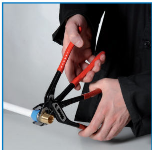
1) Отрезать трубу возле фитинга и развинтить соединение с помощью двух ключей.
